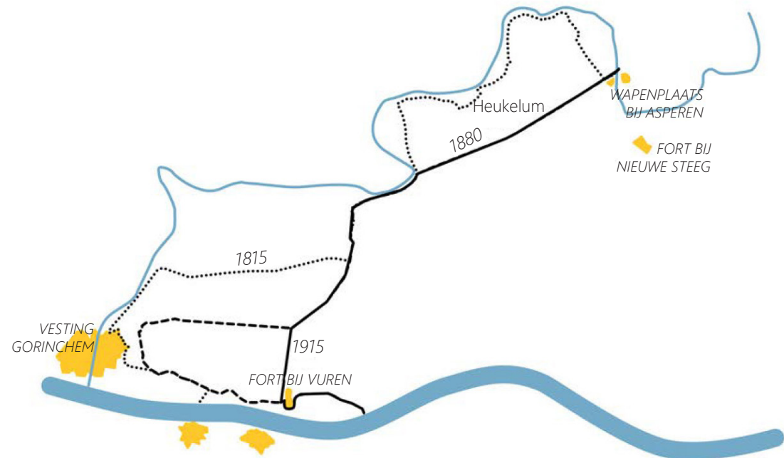
Schematische weergave van de hoofdverdedigingslijn in 1815, 1880 en 1915 (bron: Gebiedsanalyse Kernkwaliteiten Hollandse Waterlinies, Tielerwaard, Provincie Gelderland)
