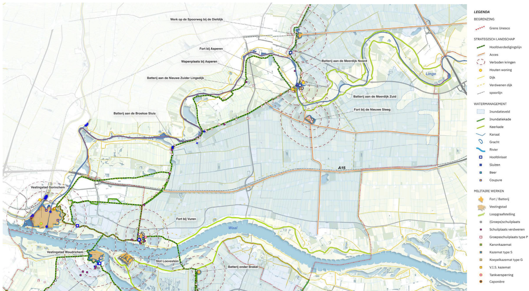
Topografische kaart met overzicht van kernkwaliteiten Tielerswaard (bron: Gebiedsanalyse Kernkwaliteiten Hollandse Waterlinies Tielerswaard, Provincie Gelderland)
